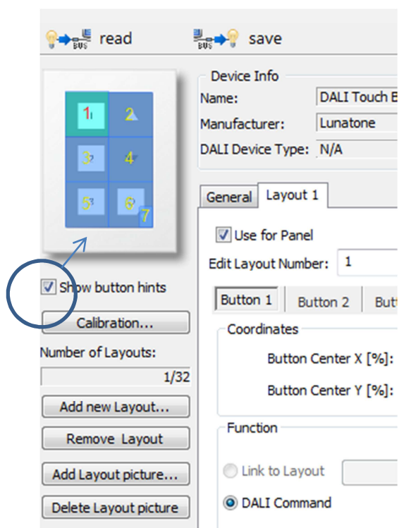
14: DALI Touch BT Module
