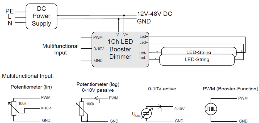
Beschaltungsvarianten
