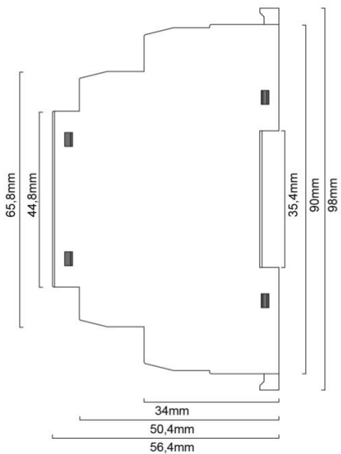
Abmessungen MC4L-HS
