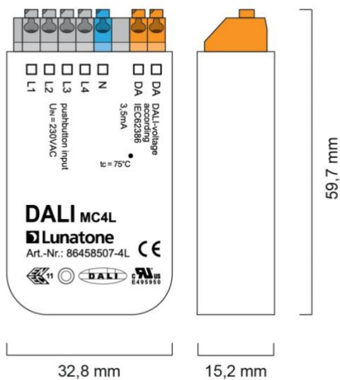
Abmessungen MC4L
