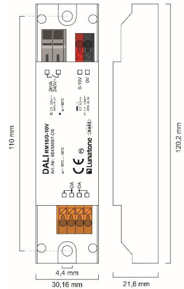
Geometrie RM16 0-10V DE
