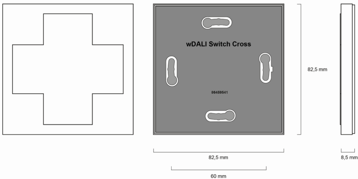
Geometrie wDALI Switch Cross (Bedieneinheit) Art.Nr.: 86459541-W (weiß RAL9010), Art.Nr.: 86459541-W16 (weiß RAL9016), Art.Nr.: 86459541-B (schwarz)
