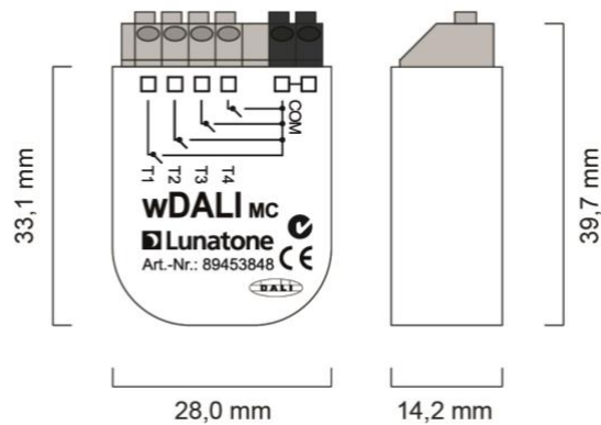
Geometrie wDALI MC (Bedieneinheit) Art.Nr.: 89453848
