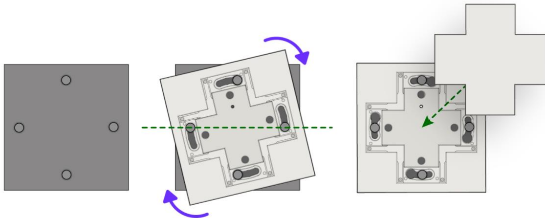
Abb.: 1.Montage anbringen 2. Schalter aufsetzen und drehen bis Schalter waagrecht ist 3. Kreuz einlegen
