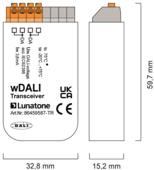
Geometrie wDALI Transceiver (Empfangseingheit) Art.Nr.: 86459587-TR
