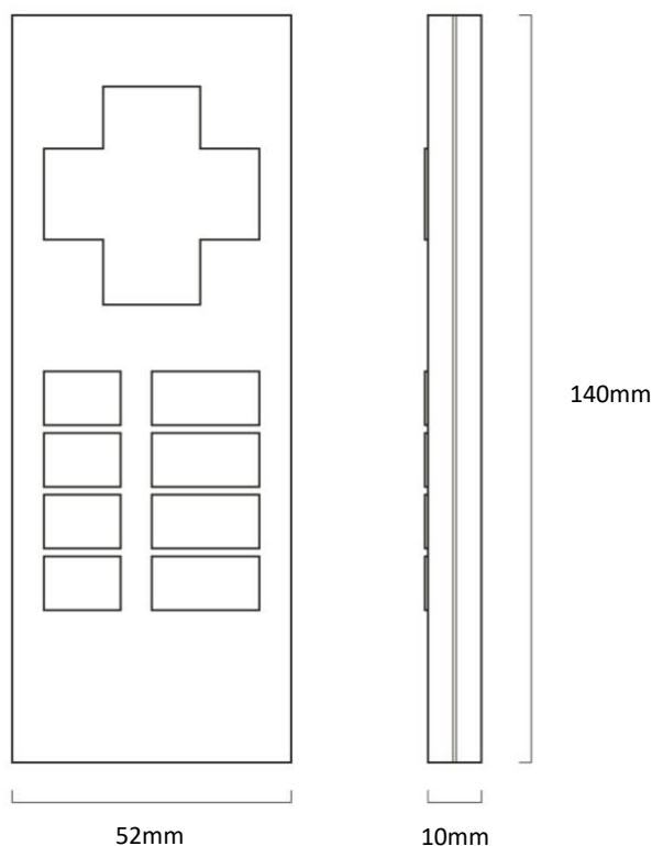
Geometrie Fernbedienung wDALI Remote (Bedieneinheit) Art.Nr.: 86459534-W (Weiß RAL9010), Art.Nr.: 86459534-B (Schwarz)
