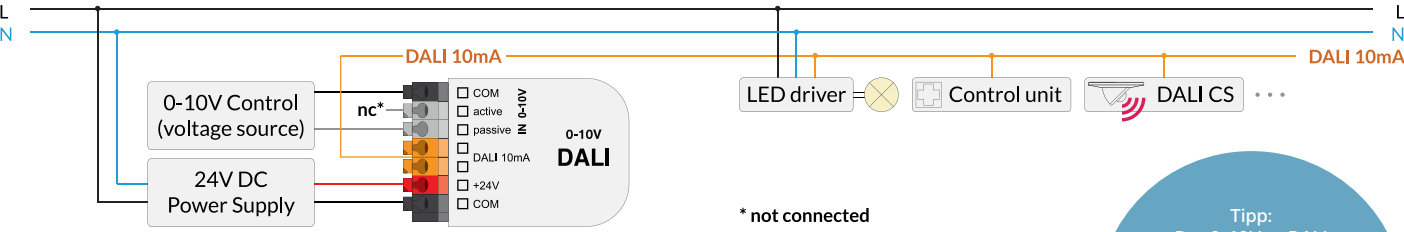
Typ. Anwendung mit 0-10V Spannung am passiven 0-10V Eingang (0-10V Steuergerät = Spannungsquelle, z.B.: SPS)
