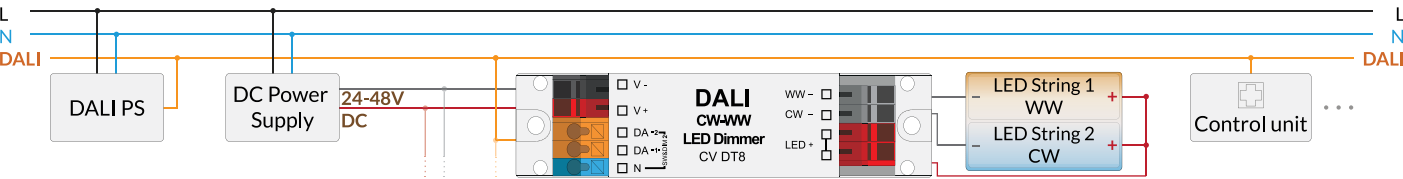
Anschlussbeispiel: CW-WW LED Dimmer CV DT8, Steuerung via DALI (SW&DIM2 Anschluss siehe Seite 2C):
