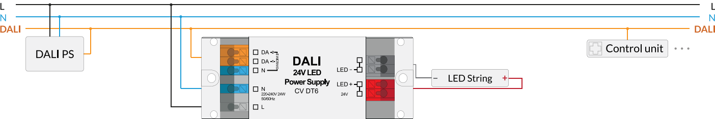
Anschlussbeispiel: DALI 24V LED Power Supply CV DT6, Steuerung via DALI (SW&DIM2 Anschluss siehe Seite 2C):
