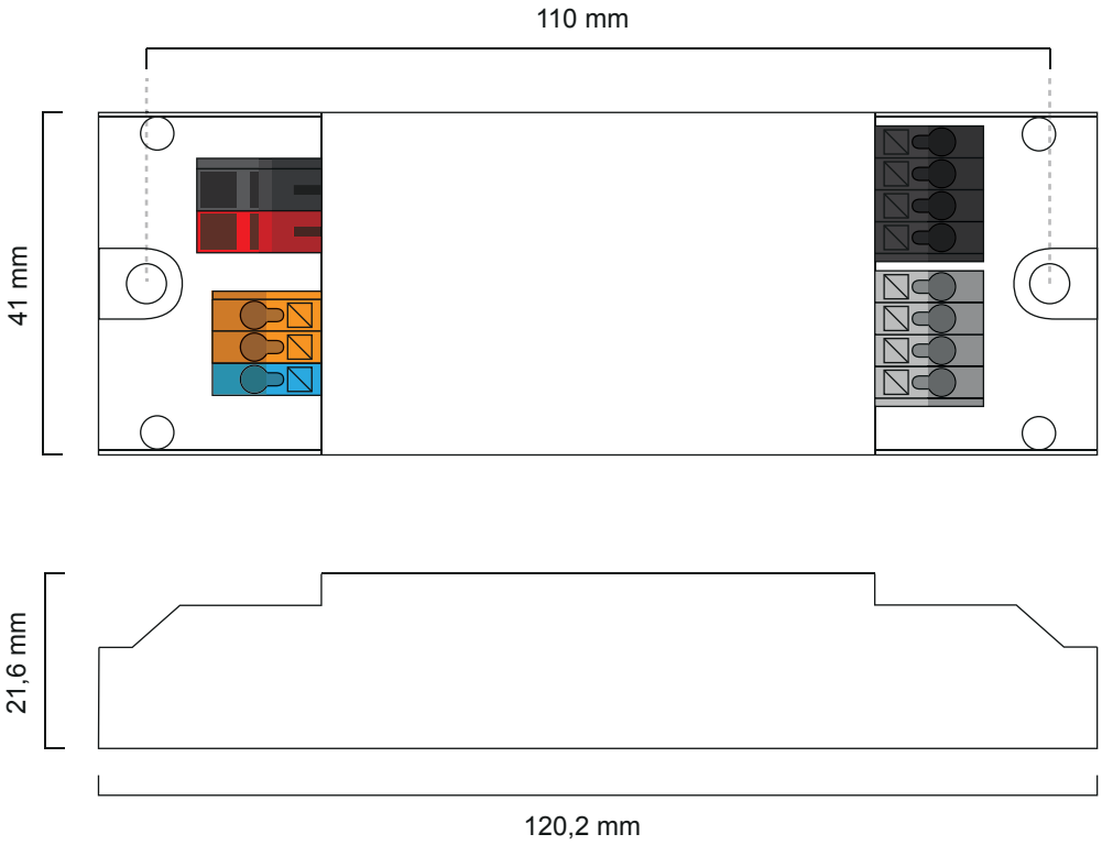
breites Deckeneinwurfgehäuse mit Zugentlastung ca. 120 × 41 × 22
