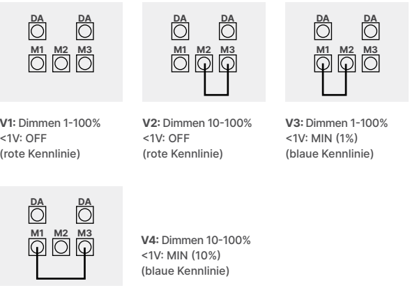
Ändern der Dimmkennlinie über Jumper durch Anschließen von entweder M1, M2, M3:
