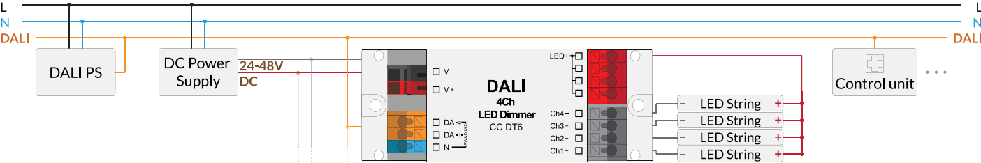
Anschlussbeispiel: 4Ch LED Dimmer CC DT6, Steuerung via DALI (SW&DIM2 Anschluss siehe Seite 2C):
