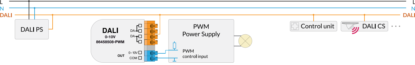
86458508-PWM ermöglicht das Einbinden von elektrischen Geräten mit PWM Steuereingang.
