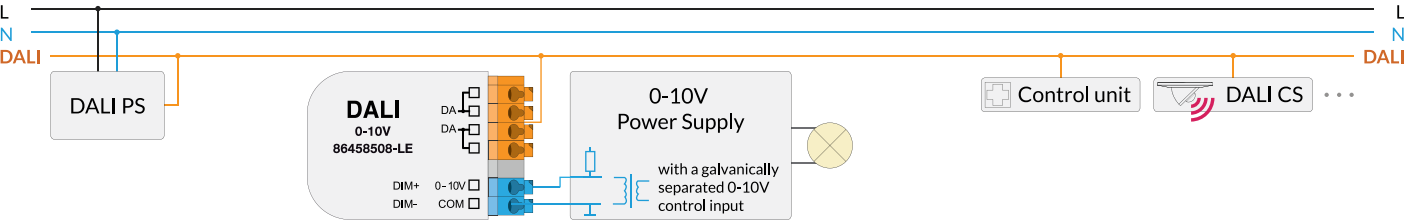
86458508-LE ermöglicht das Einbinden von elektrischen Geräten mit internem galvanisch getrenntem 0 bzw. 1-10V Steuereingang.
