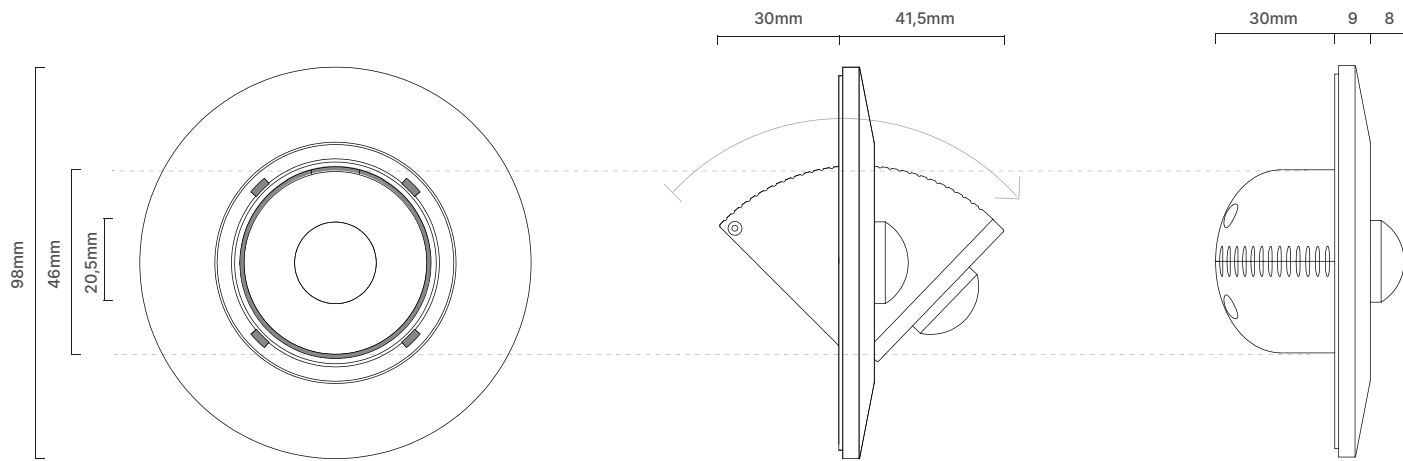
Masszeichnung des DALI CS & DALI LS (Standard Version, zur direkten Montage in Installationsdosen/ Hohlraumwänden)
