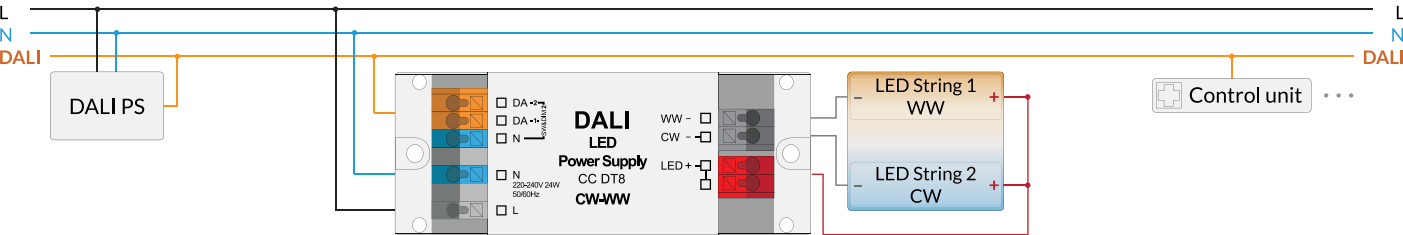
Anschlussbeispiel: DALI LED Power Supply CW-WW CC DT8, Steuerung via DALI (SW&DIM2 Anschluss siehe Seite 2C):
