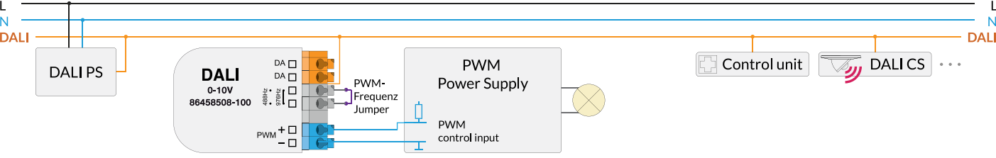
86458508-100 ermöglicht das Einbinden von bis zu 100 elektrischen Geräten mit PWM Steuereingang.
