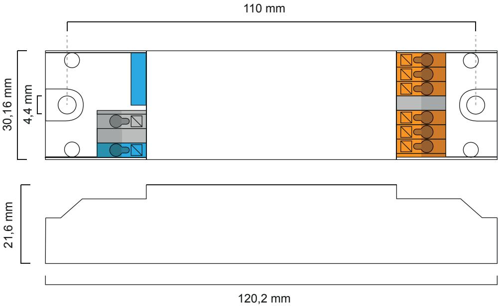
schmales Deckeneinwurfgehäuse mit Zugentlastung ca. 120 × 30 × 22
