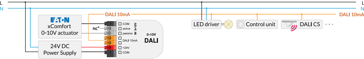
Beispiel: Steuerung von DALI Leuchten mit z.B. xComfort von EATON
