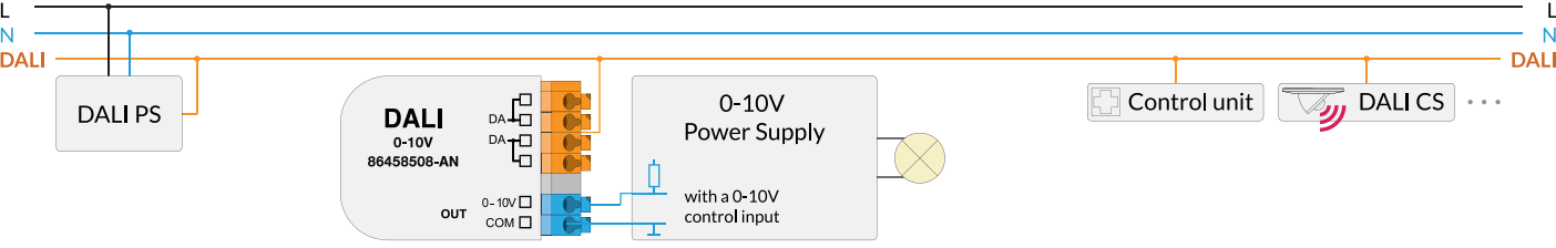
86458508-AN ermöglicht das Einbinden von elektrischen Geräten mit 0 bzw. 1-10V Steuereingang.
