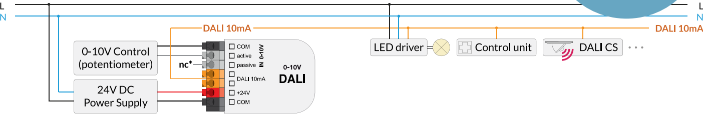
Typ. Anwendung mit 100k Potentiometer am aktiven 0-10V Eingang (0-10V Steuergerät = Verbraucher)
