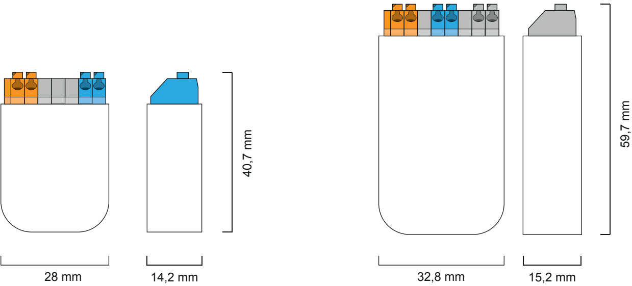
kleines Dosengehäuse ca. 40 × 28 × 15 Das kompakte Gerät kann in die Unterputzdose hinter dem Schalter eingelegt werden.
