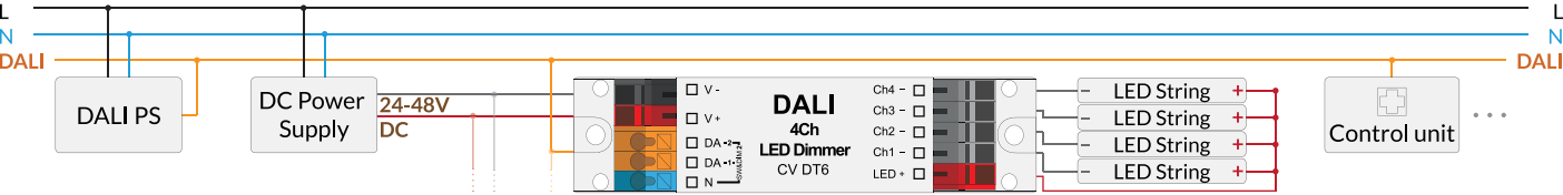
Anschlussbeispiel: 4Ch LED Dimmer CV DT6, Steuerung via DALI (SW&DIM2 Anschluss siehe Seite 2C):
