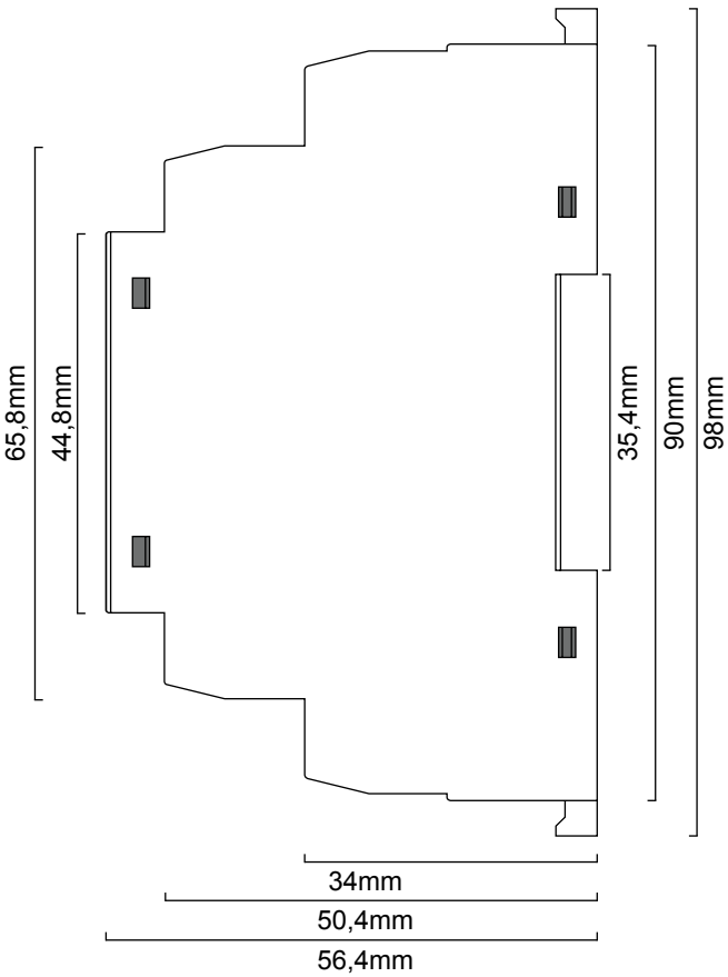
1TE Hutschienengehäuse ca. 98 × 17,5 × 57 für den Schaltscharnk
