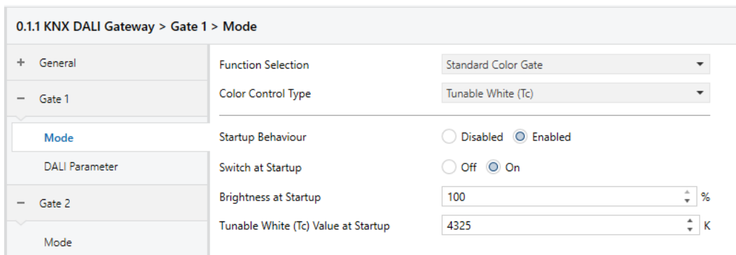
Abb.9 Gate Einstellungen ETS: Tab „Mode“ Standard Color Gate für Tunable White
