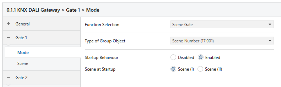
Abb.11 Gate Einstellungen ETS: Beispiel Standard Scene Gate
