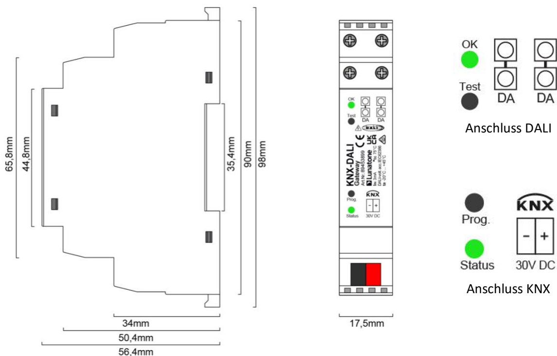
Abmessungen KNX-DALI Gateway Art.Nr.: 89453899
