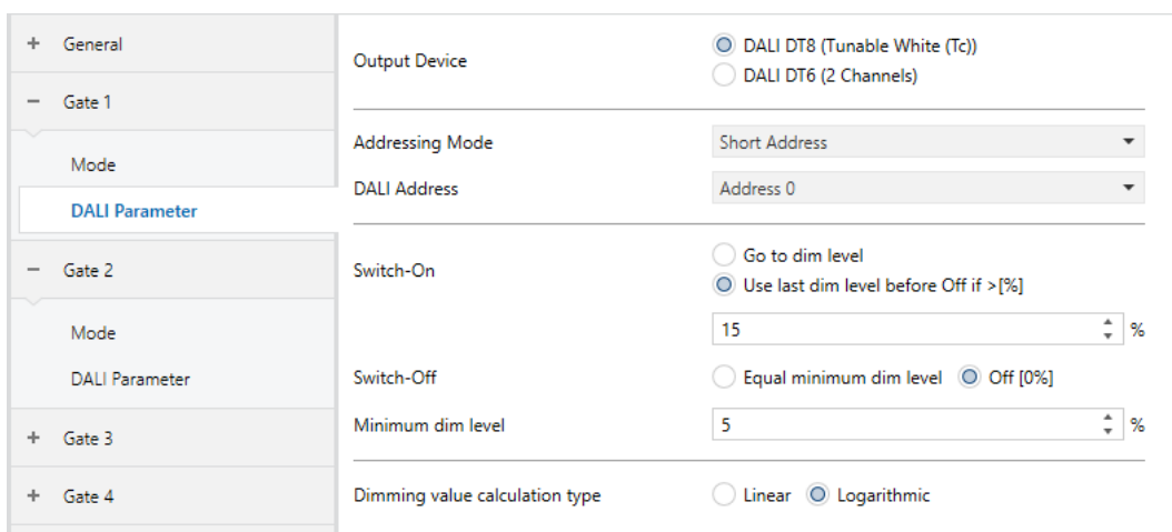
Abb.10 Gate Einstellungen ETS: Tab „DALI Parameter“ Standard Color Gate
