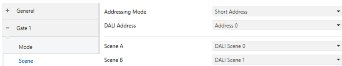
Abb.12 Gate Einstellungen ETS: Beispiel Standard Scene Gate
