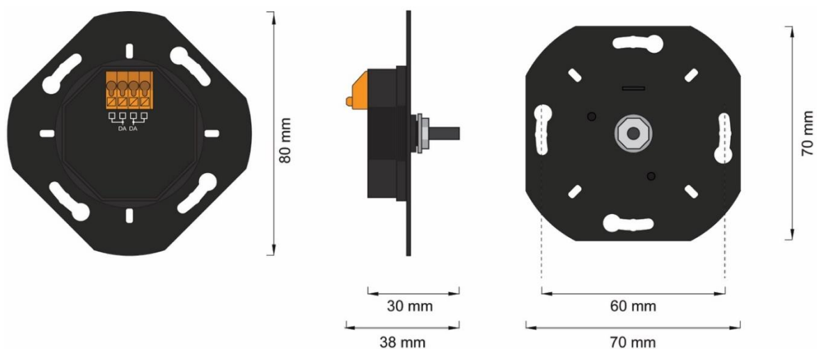
Abmessungen Drehschalter
