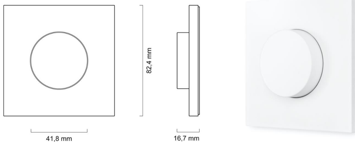
Abmessungen Drehschalter
