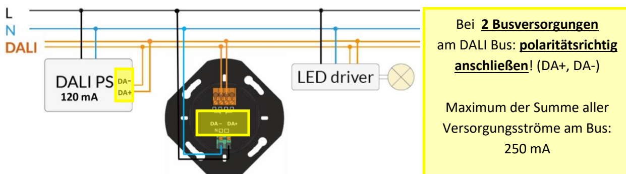
Abb. 1 DALI-2 ROT PS – Beispielinstallation mit zweiter DALI PS am DALI Bus
