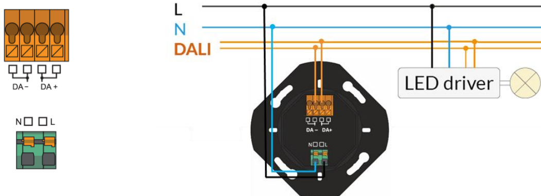
Anschlussplan DALI-2 ROT Touch PS
