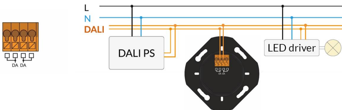
Anschlussplan DALI-2 ROT
