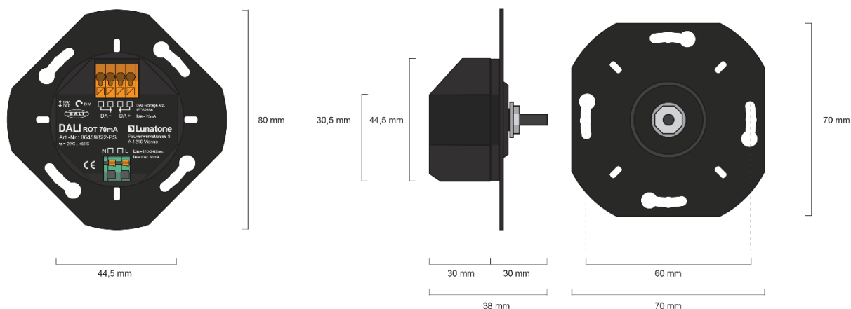
Abmessungen DALI-2 ROT Touch PS
