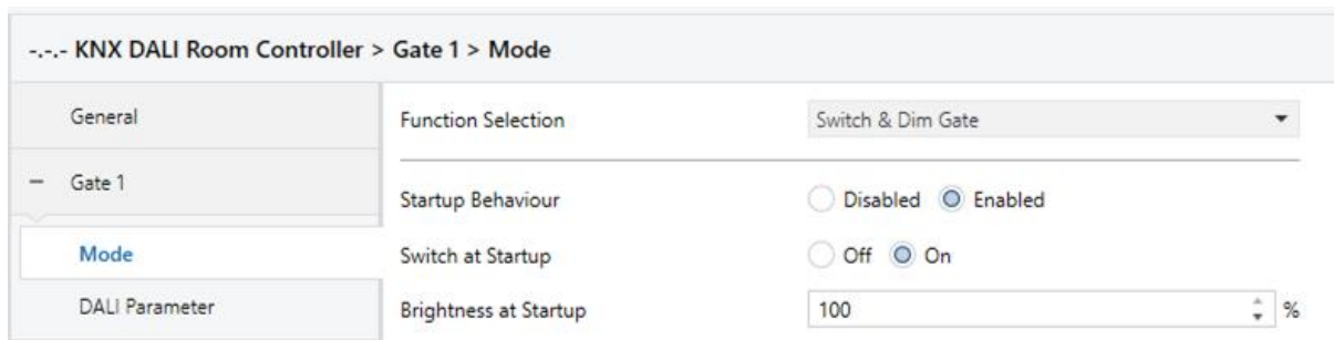
Fig.5 Gate Settings ETS: Tab „Mode“ Switch & Dim Gate
