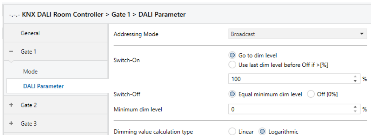
Abb.6 Gate Settings ETS: Tab „DALI Parameter“ Switch & Dim Gate
