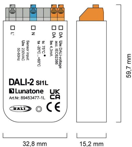
Abmessungen DALI SI 1L
