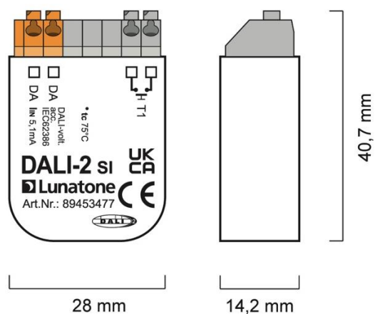
Abmessungen DALI SI
