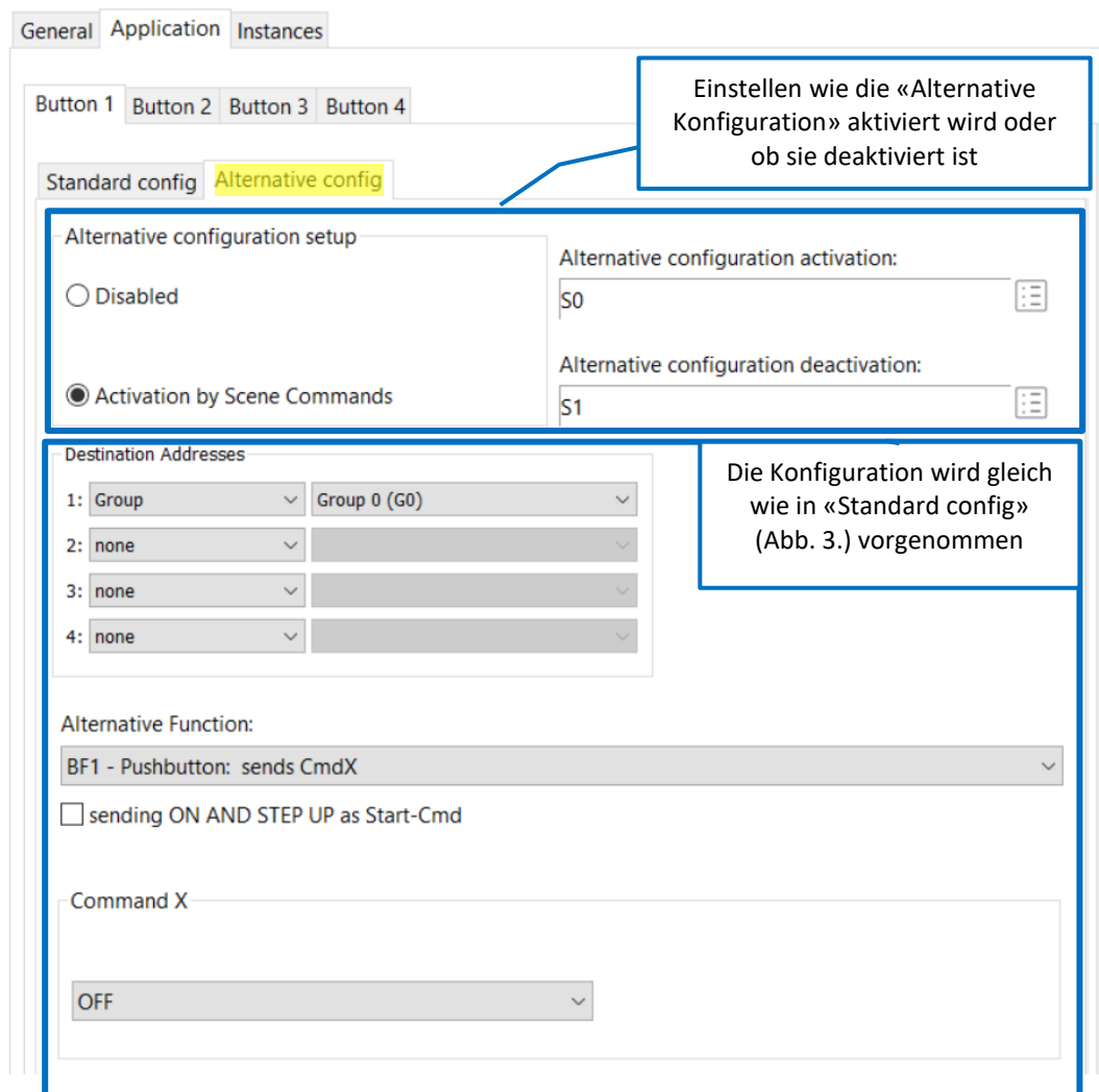
Abb. 11.: Cockpit Einstellung: Alternative Konfiguration
