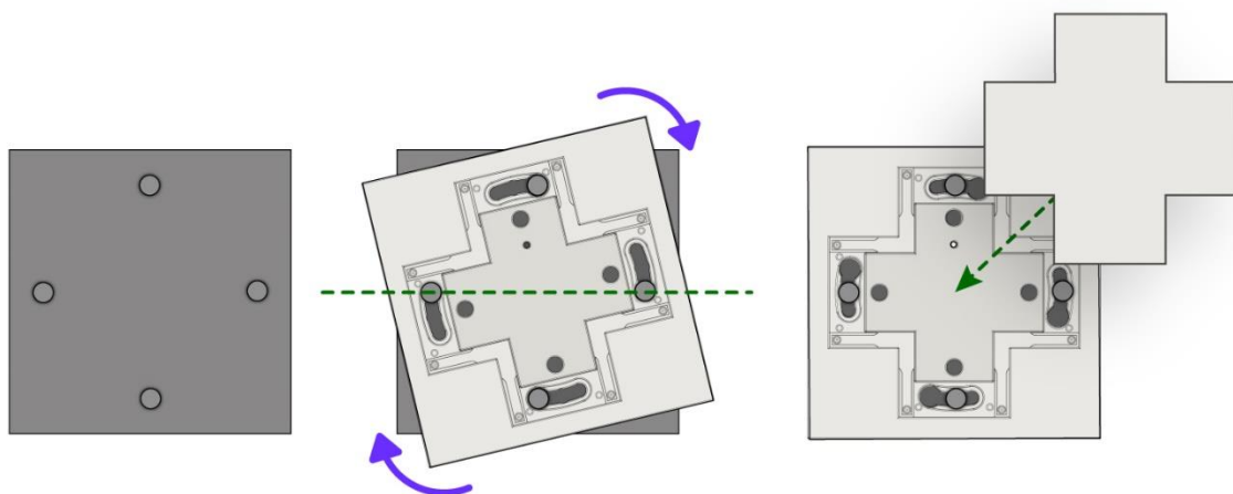
Abb. 3.: 1.Montage anbringen 2. Schalter aufsetzen und drehen bis Schalter waagrecht ist 3. Kreuz einlegen
