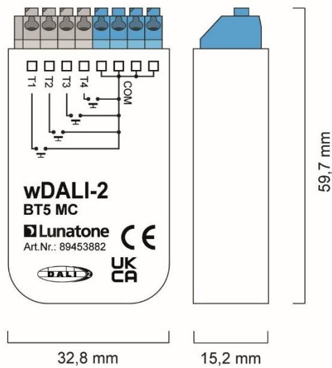
Geometrie wDALI-2 BT5 MC
