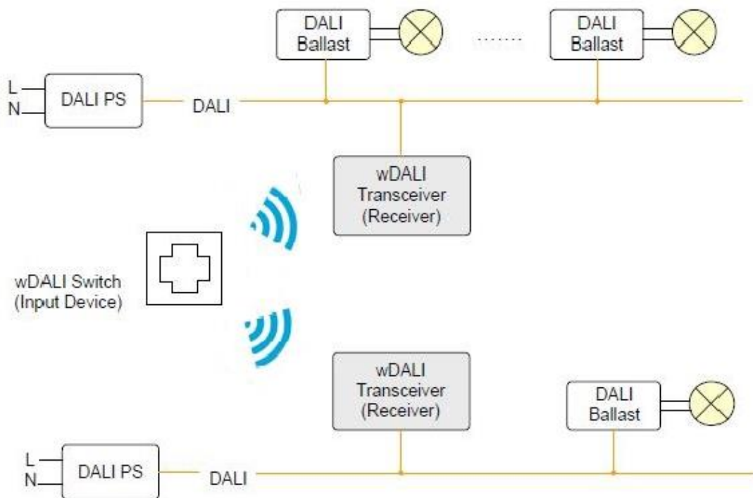
Abb. 2 typische Anwendung: drahtlose Steuerung ein Bediengerät, gleichzeitige Bedienung mehrerer DALI-Kreise
