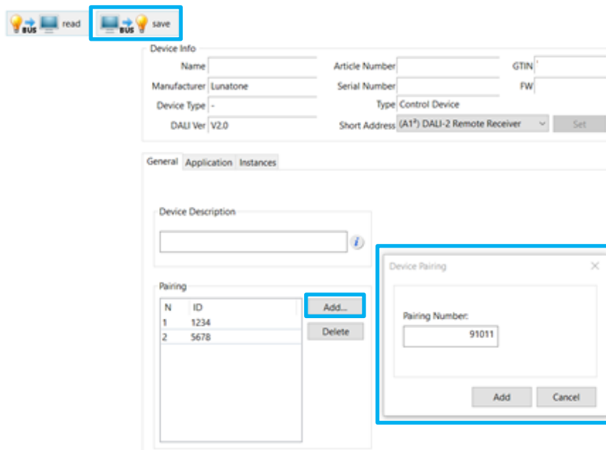
Abb. 4.: Koppeln von Steuergerät und Receiver
