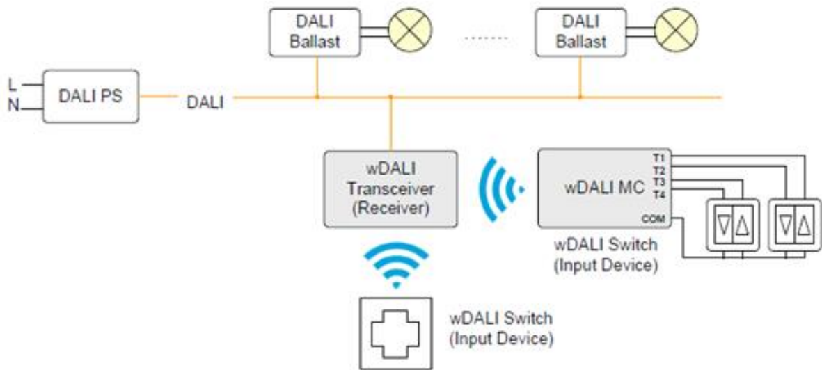
Abb. 1 typische Anwendung: drahtlose Steuerung: mehrere Bediengeräte, ein Empfänger
