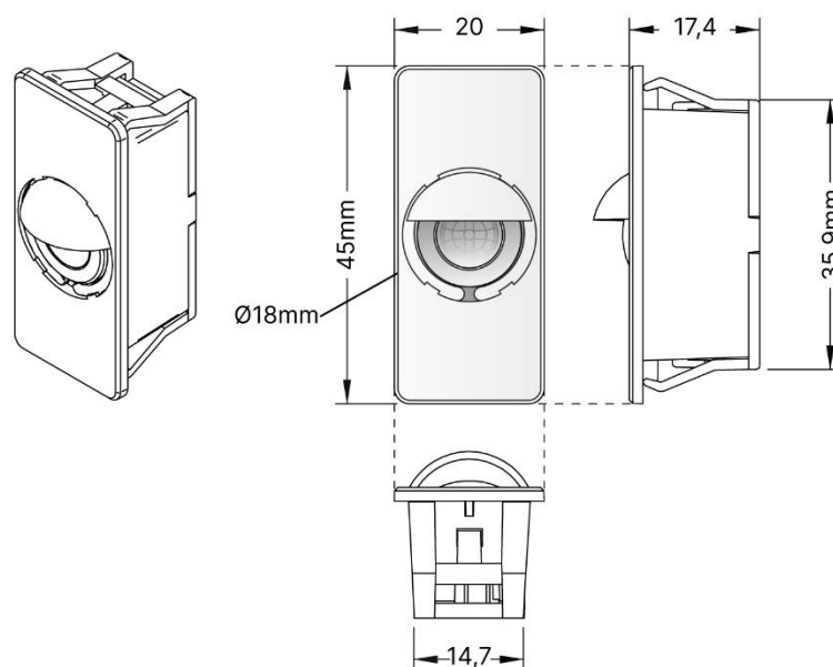
Abmessungen und Platzbedarf – Leuchteneinbau - DALI-2 CS 2045 - 86451485-LA-W16
