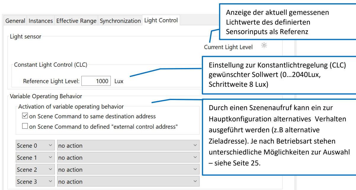
Abb. 14 Reiter: „Licht Regelung“ – Betriebsart: Konstantlichtregelung
