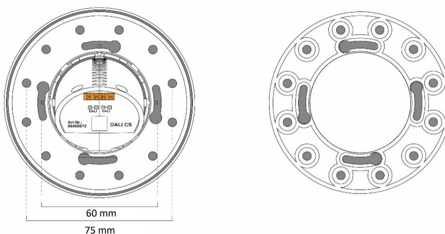
Abmessungen Montagering
