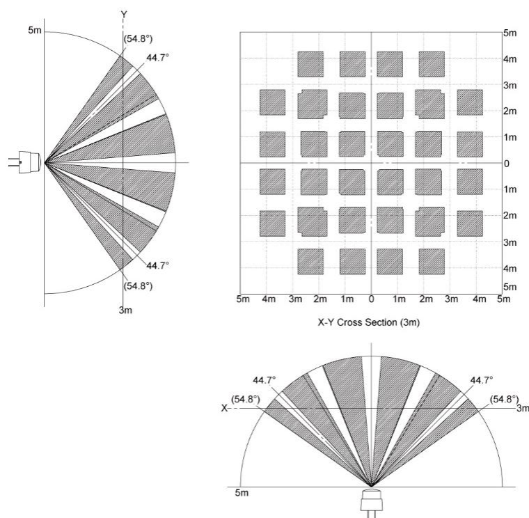
Abb. 7 CS-LE/-LA Leuchteineinbau Bewegungserkennung (Artikelnummern: 86451485-LA-W16) Erfassungsbereich: X-Y-Querschnitt bei 3m.
